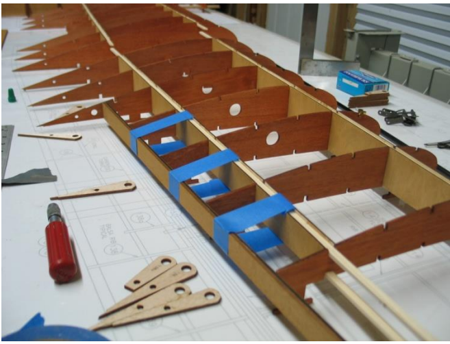
Secure aileron leading edge
